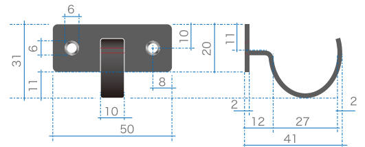
ZNB0003 のれん受け-正面付け-KK (黒 艶消し) 【製品サイズ】 横50mm×縦31mm×奥行き41mm
