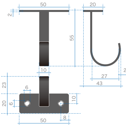
ZNB0005 のれん受け-天井付け-KK (黒 艶消し) 【製品サイズ】 横50mm×縦55mm×奥行き43mm
