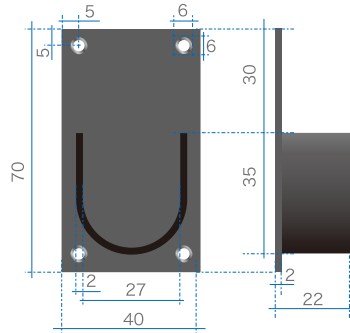
ZNB0004 のれん受け-枠内付け-KK (黒 艶消し) 【製品サイズ】 横40mm×縦70mm×奥行き22mm
